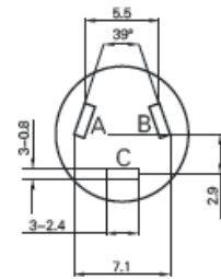
引线脚分布图
